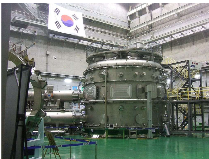
Obrázek 6 - jihokorejský tokamak KSTAR, držitel rekordu v délce běhu na jedno spuštění (zdroj: wikipedia.org)
